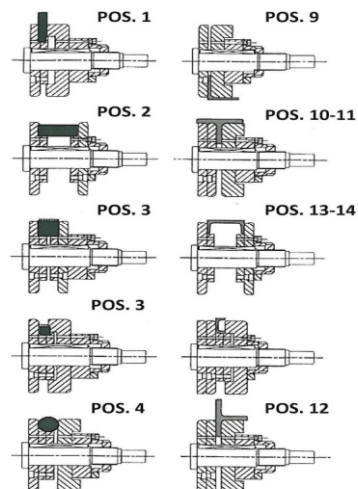
schemat montażu rolek dla różnych przekrojów
